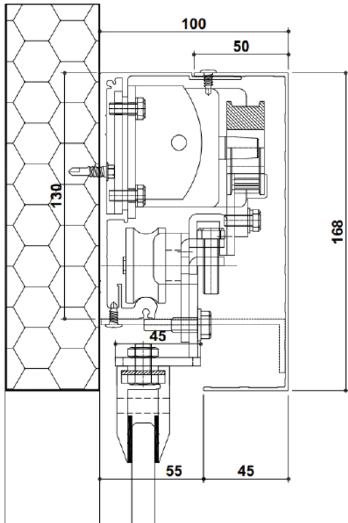
Mặt cắt hộp kỹ thuật
